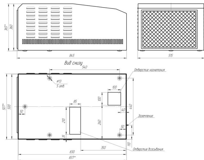
Габаритные и установочные размеры кондиционера КТА-01.
